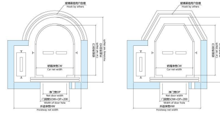
井道平面布置图 Hoistway plan layout
